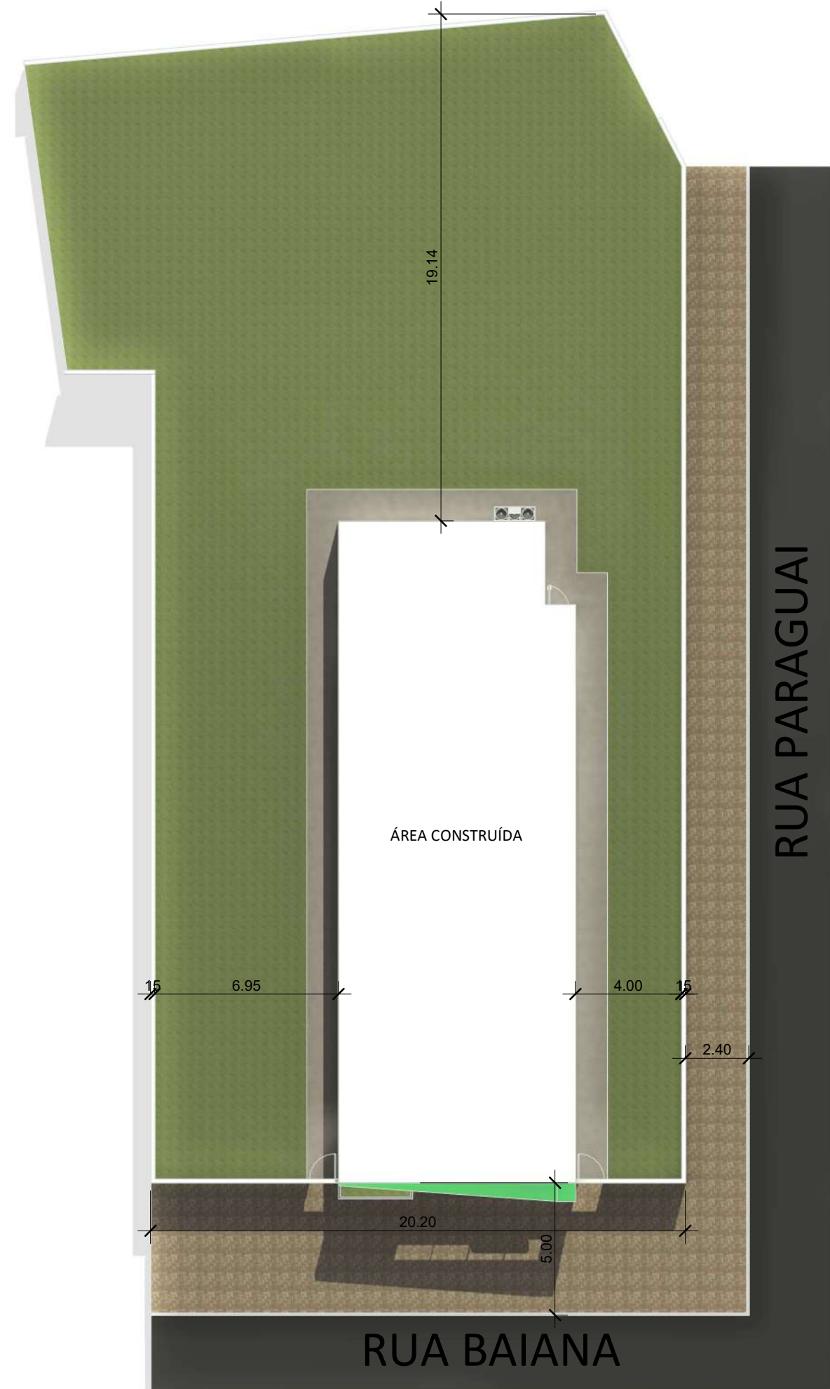
6 PLANTA DE LOCAÇÃO 1 : 200
