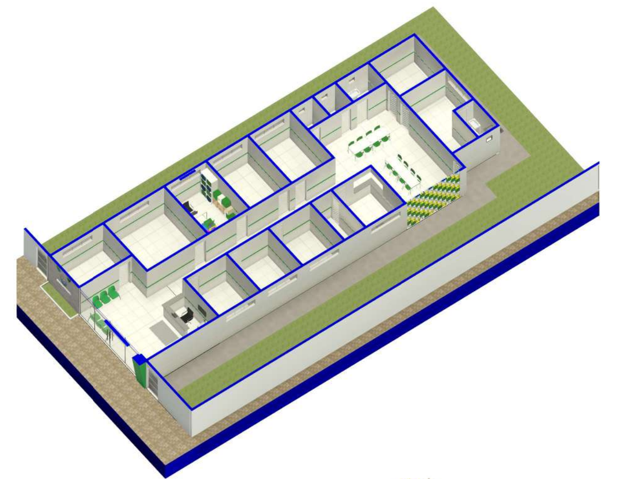
11 CORTE ISOMÉTRICO 01
