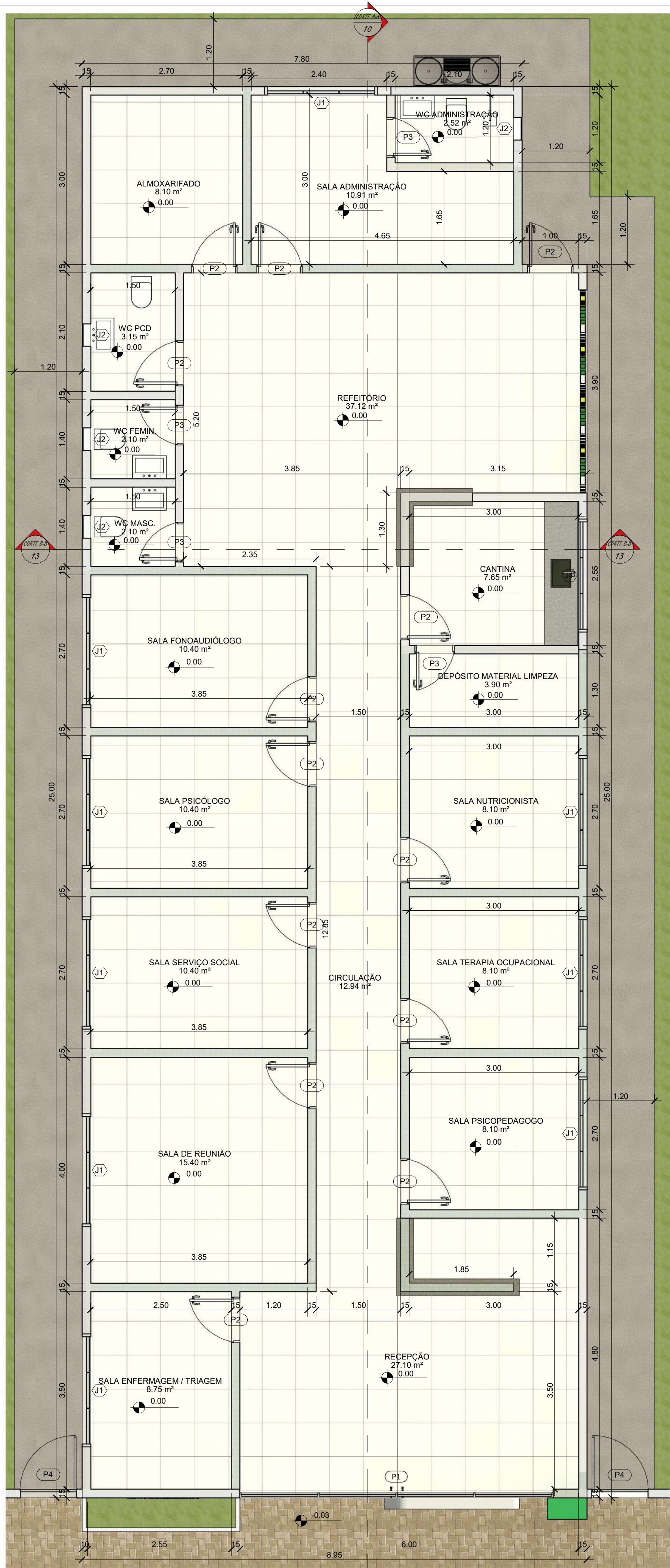
1 PLANTA BAIXA 1 : 50
