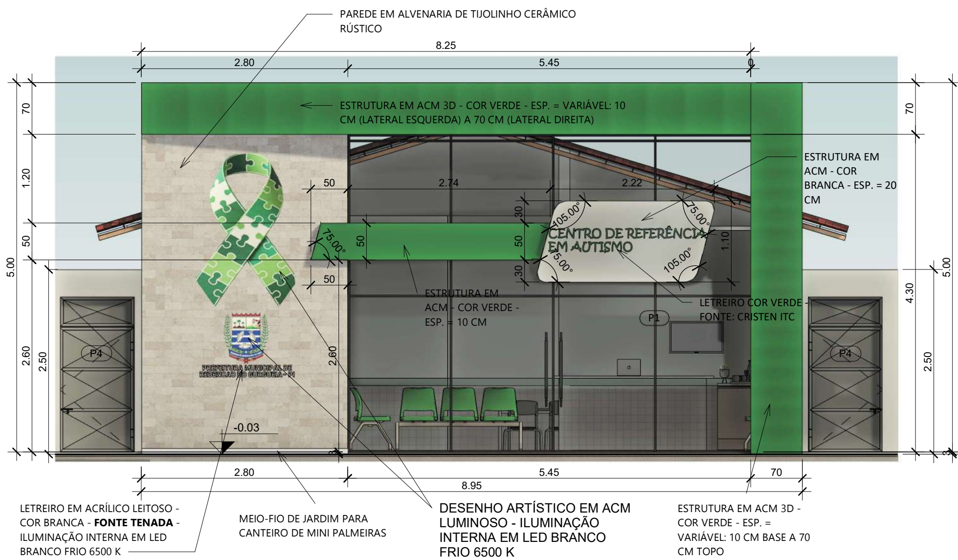
2 FACHADA 1 : 50
