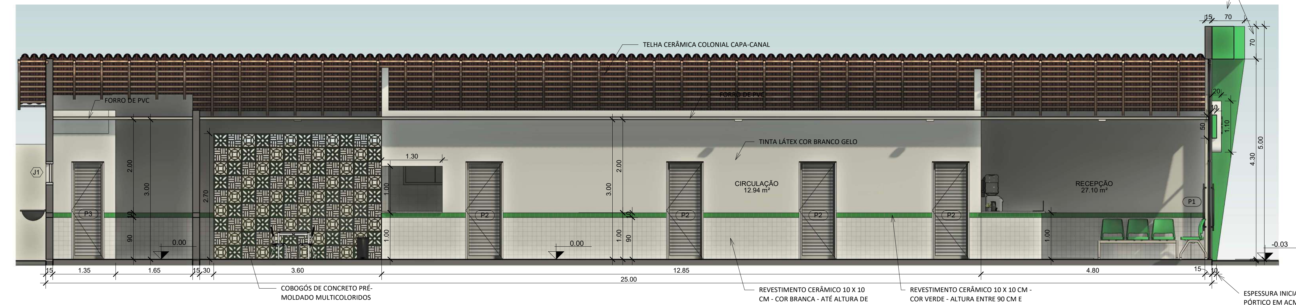
10 CORTE A-A 1 : 50
