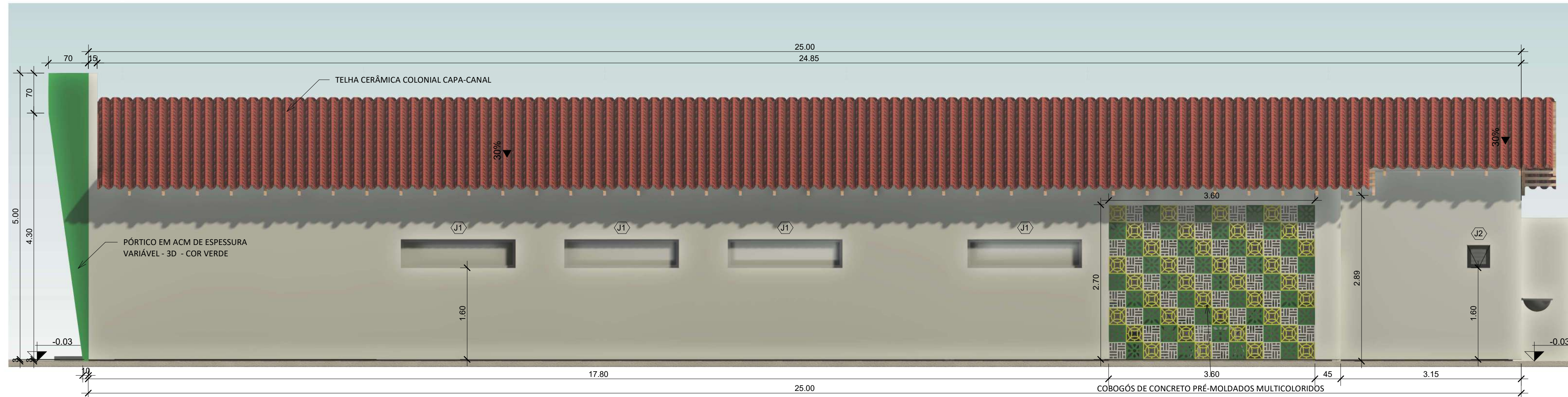
8 LATERAL DIREITA 1 : 50
