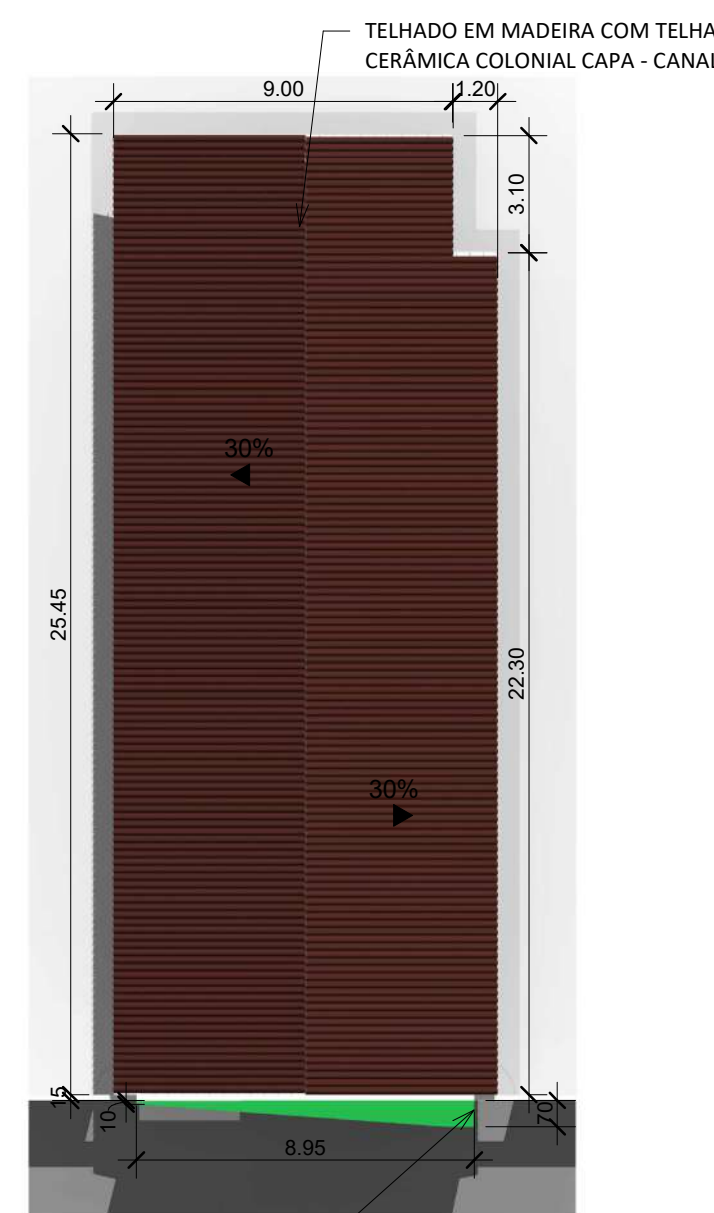
7 PLANTA COBERTURA 1 : 200
