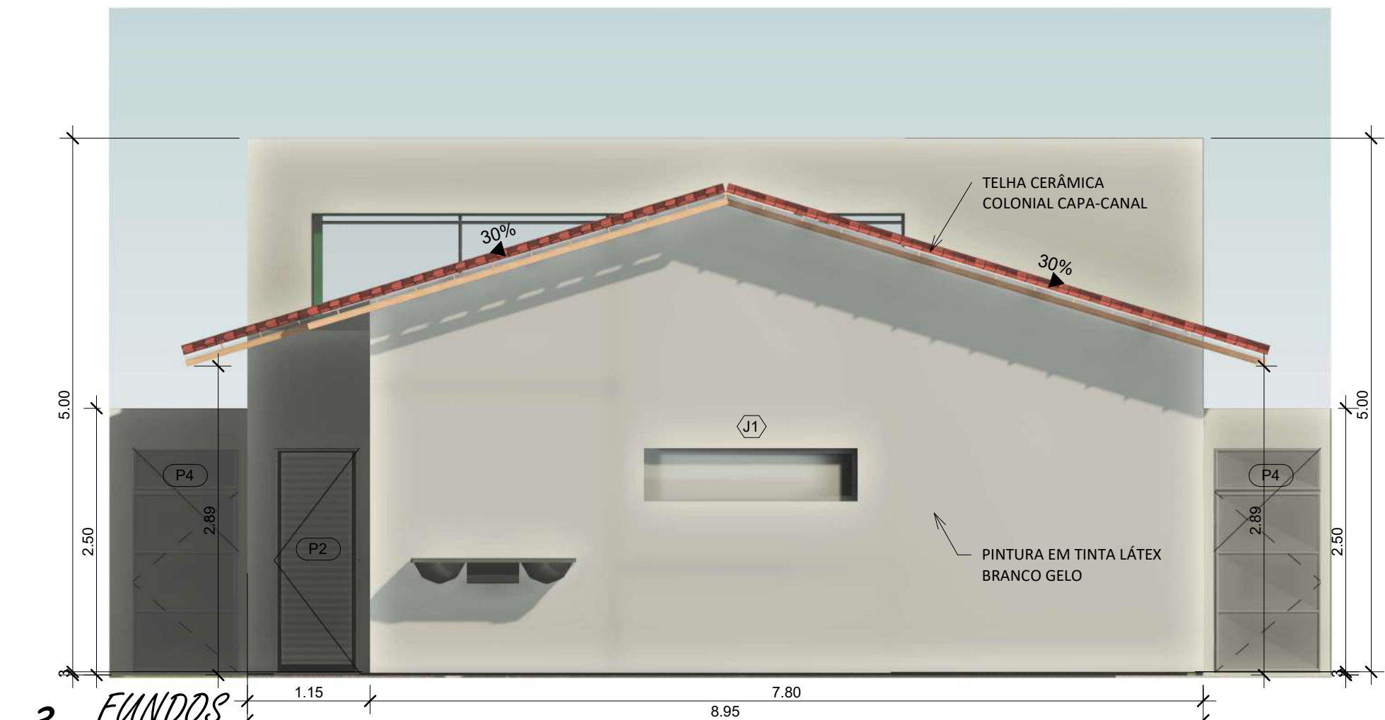
3 FUNDOS 1 : 50
